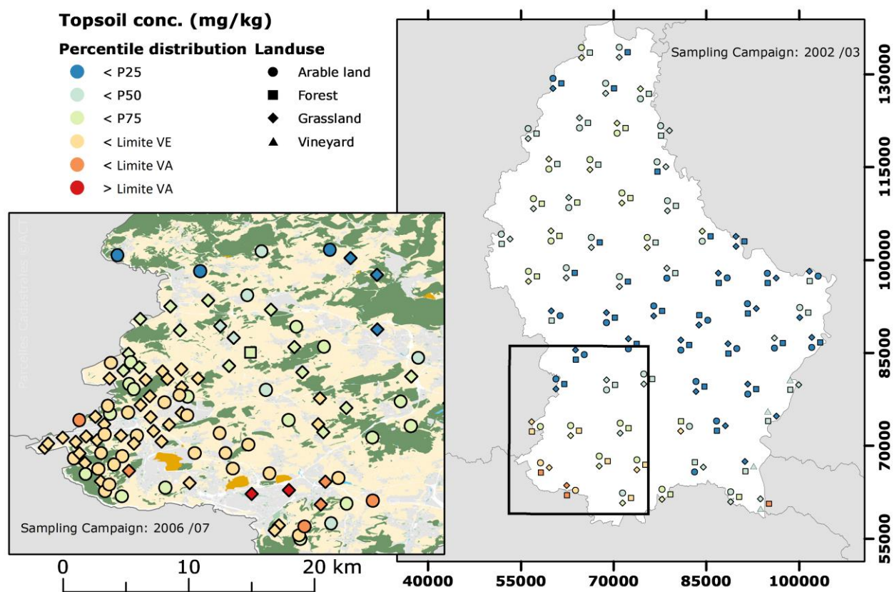
Figure 27. Représentation spatiale des concentrations quasi-totales en zinc des sols de surface au Grand-Duché de Luxembourg. La représentation reprend les résultats de deux campagnes d'échantillonnage, une à échelle nationale (2002/03) et une à échelle régionale (2006/07).
