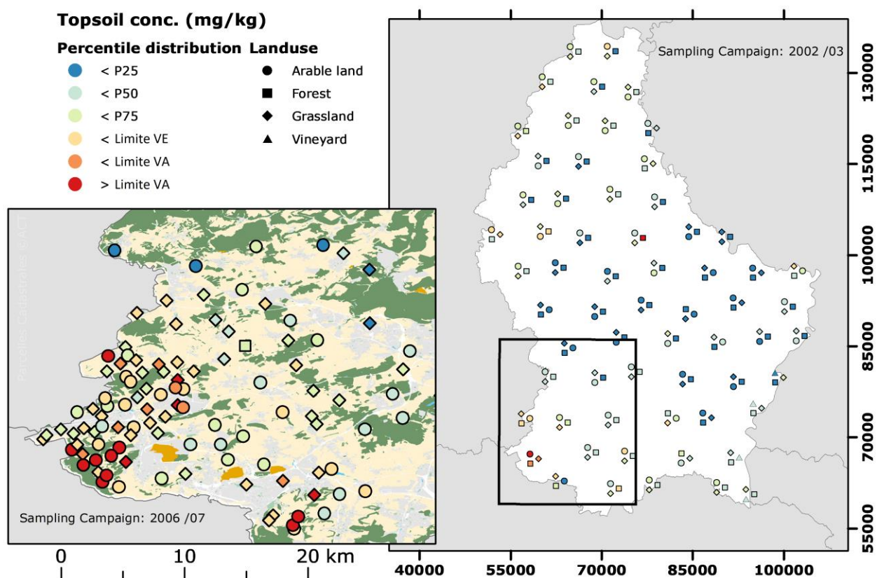
Figure 8. Représentation spatiale des concentrations quasi-totales en chrome des sols de surface au Grand-Duché de Luxembourg. La représentation reprend les résultats de deux campagnes d'échantillonnage, une à échelle nationale (2002/03) et une à échelle régionale (2006/07).
