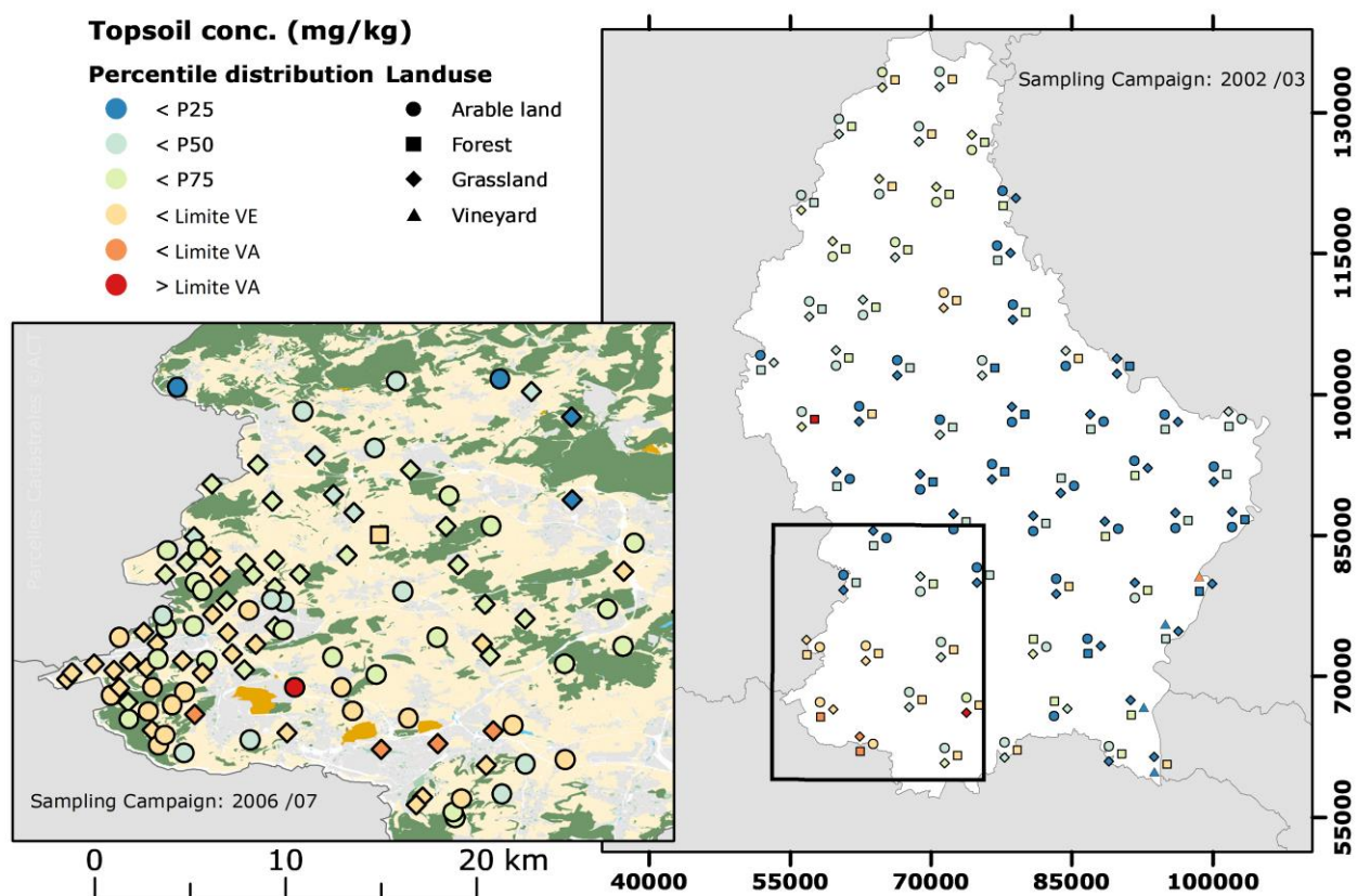
Figure 23. Représentation spatiale des concentrations quasi-totales en plomb des sols de surface au Grand-Duché de Luxembourg. La représentation reprend les résultats de deux campagnes d'échantillonnage, une à échelle nationale (2002/03) et une à échelle régionale (2006/07).
