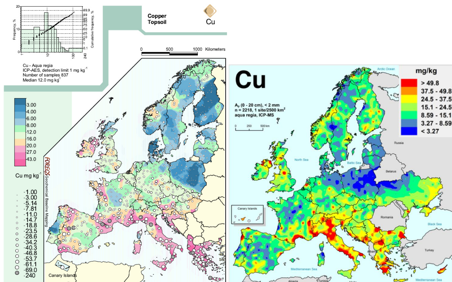
Figure 13. Cartes des concentrations en cuivre dans les sols de surface en Europe. À gauche : données FORGES (De Vos et al., 2006). À droite : données GEMAS (Reimann et al., 2014).
