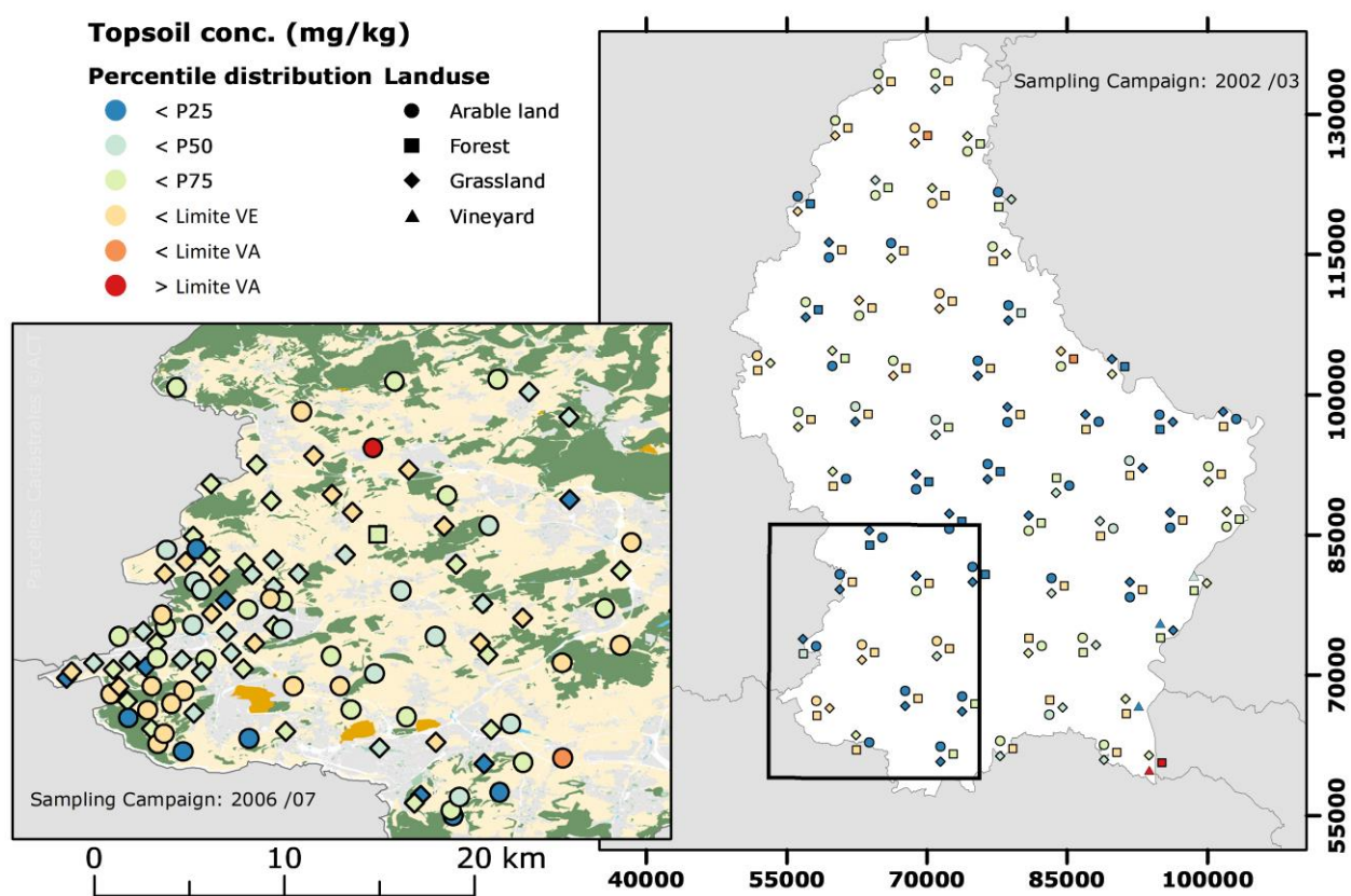
Figure 17. Représentation spatiale des concentrations quasi-totales en mercure des sols de surface au Grand-Duché de Luxembourg. La représentation reprend les résultats de deux campagnes d'échantillonnage, une à échelle nationale (2002/03) et une à échelle régionale (2006/07).
