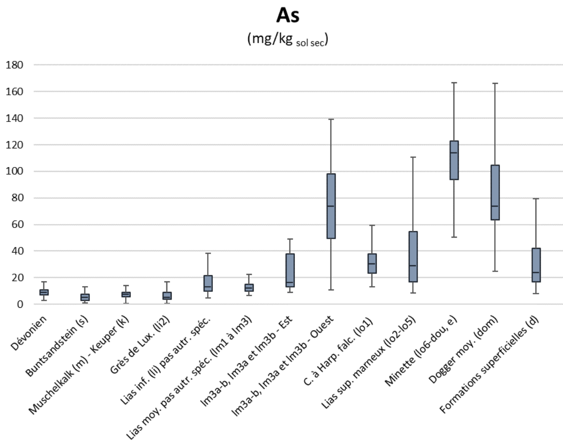
Figure 4. « Box and Whisker plot » des CF quasi-totales en arsenic en mg/kg sol sec distingué selon les régions homogènes géologiques.
