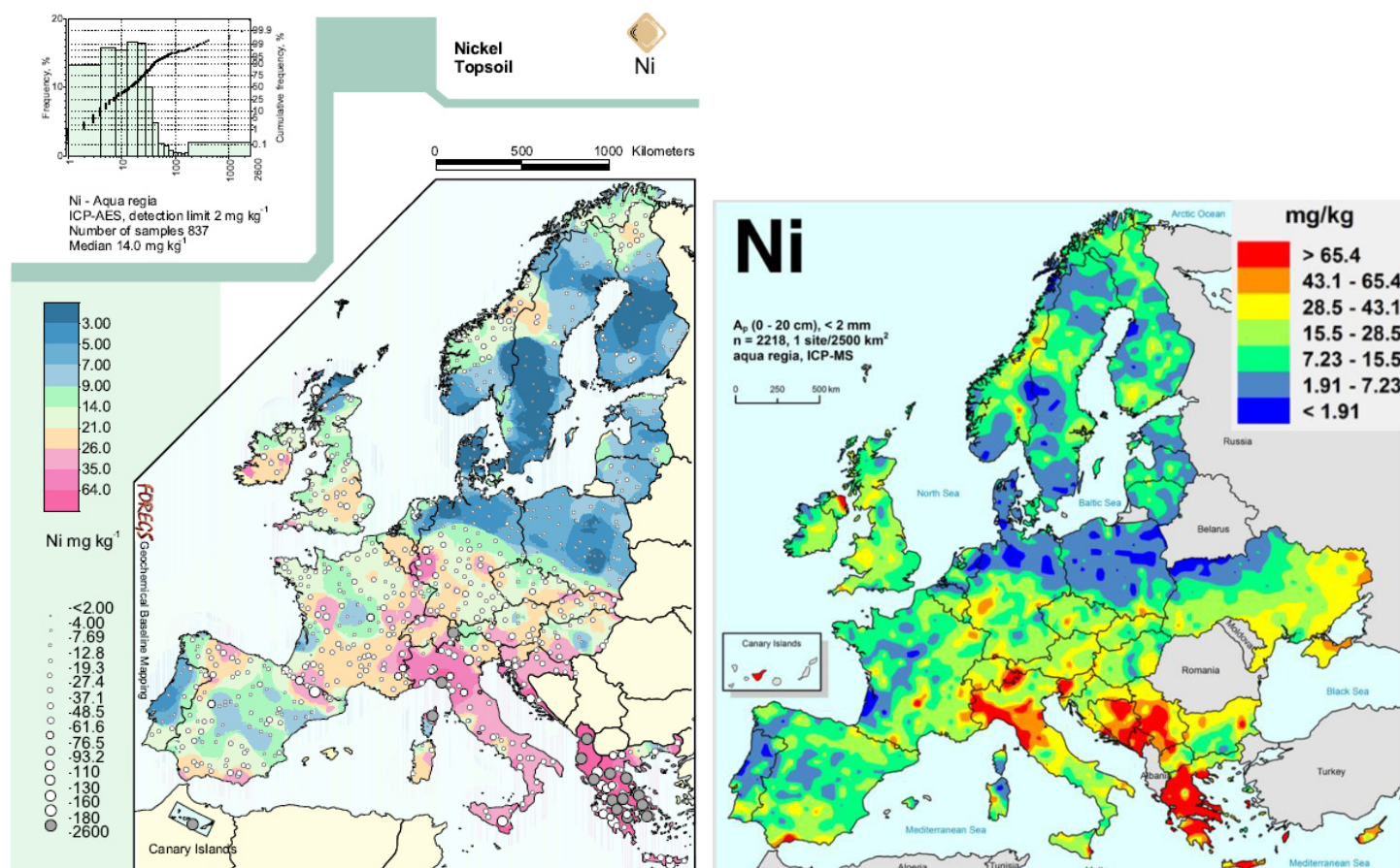
Figure 19. Cartes des concentrations en nickel dans les sols de surface en Europe. À gauche : données FORGES (De Vos et al., 2006). À droite : données GEMAS (Reimann et al., 2014).
