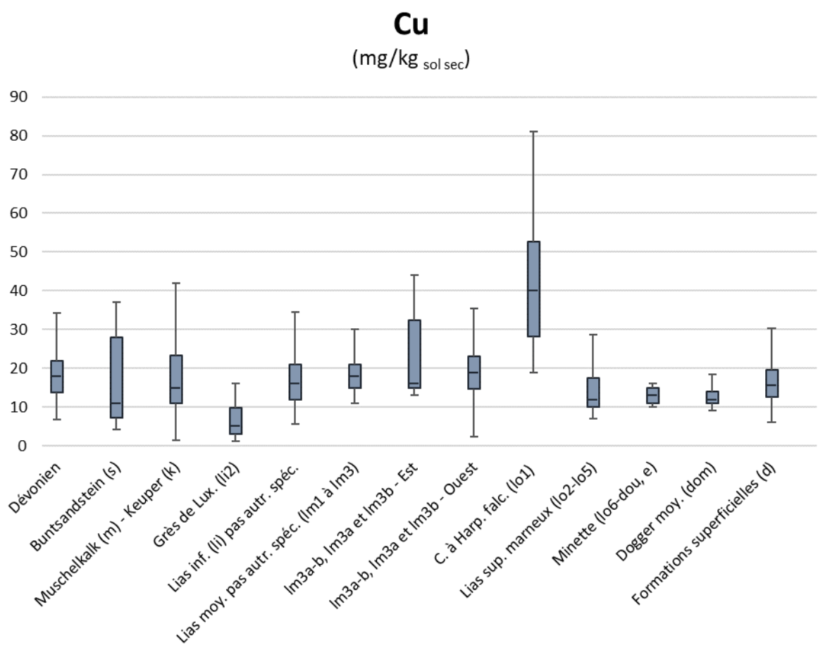
Figure 15. « Box and Whisker plot » des CF quasi-totales en cuivre en mg/kg sol sec distinguées selon les régions homogènes géologiques.
